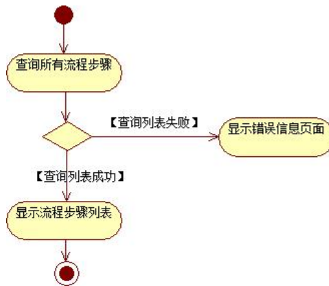
图 3.4.3 流程步骤信息列表活动图
