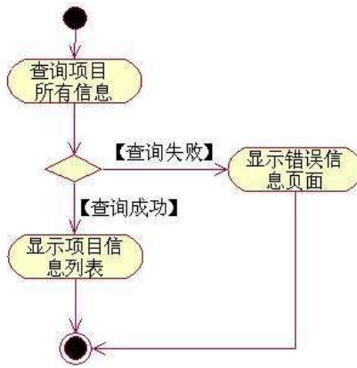
图 3.1.4 项目信息列表活动图
