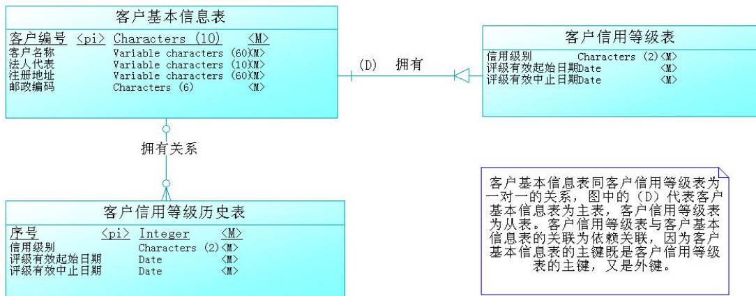
图 2.10.2 逻辑数据模型
