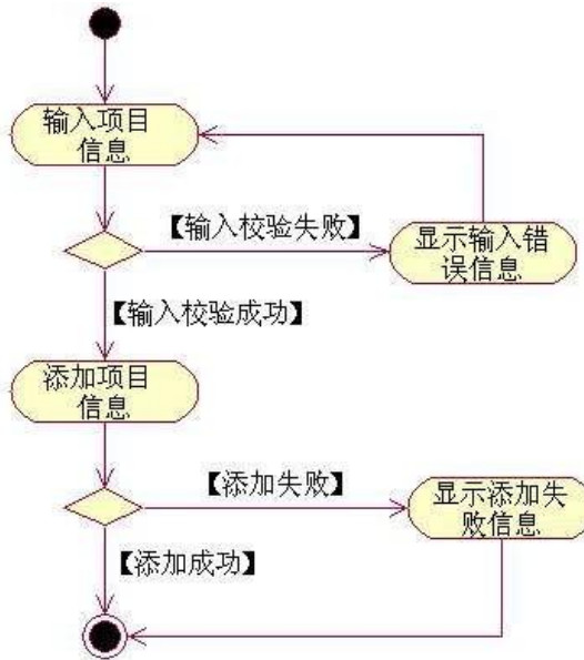
图3.1.5 添加项目信息活动图
