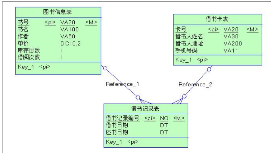
图 2.5.2 逻辑数据模型
