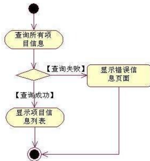
图 3.3.4 招标项目信息列表活动图
