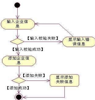
图1.2.5 添加企业信息活动图
