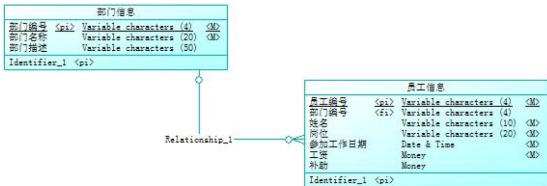
图 2.10.2 逻辑数据模型
