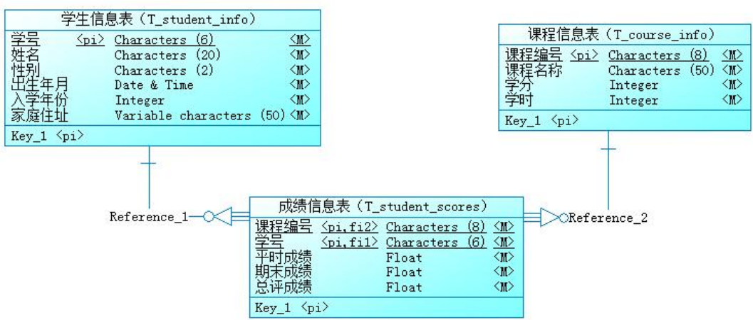
图 2.4.2 逻辑数据模型
