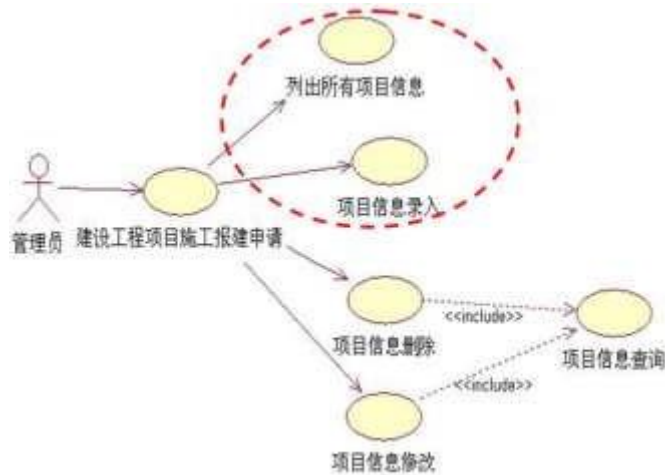
图 3.1.3 建设工程项目施工报建申请模块用例图
