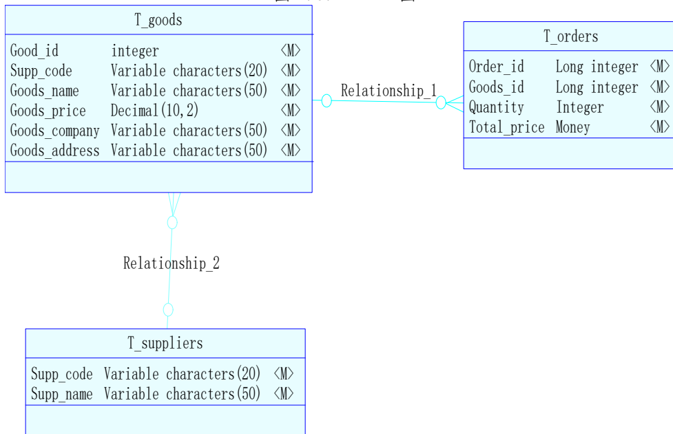
图 2.9.2 逻辑数据模型
