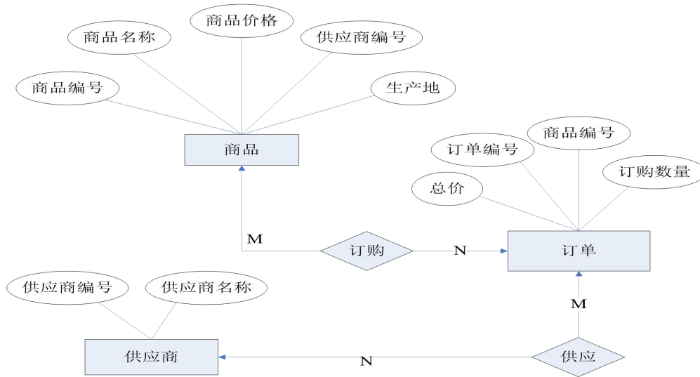
图 2.9.1 E-R 图
