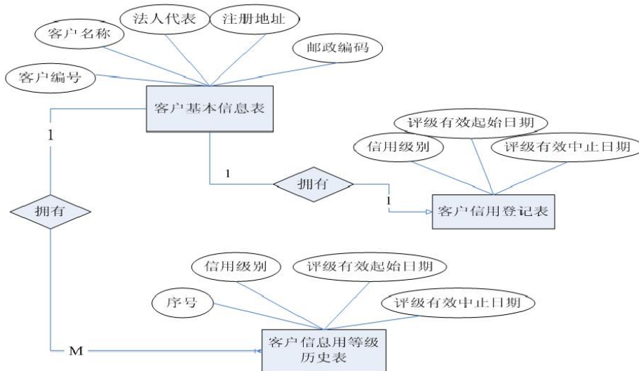
图 2.10.1 E-R 图
