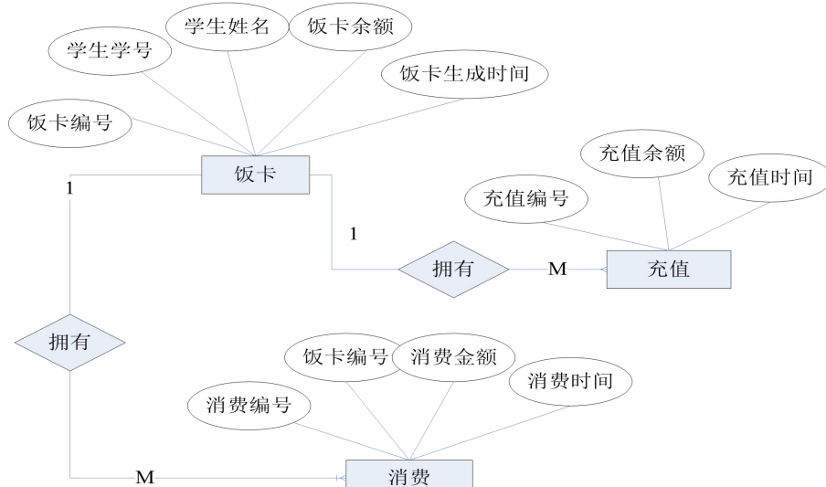
图 2.6.1 E-R 图
