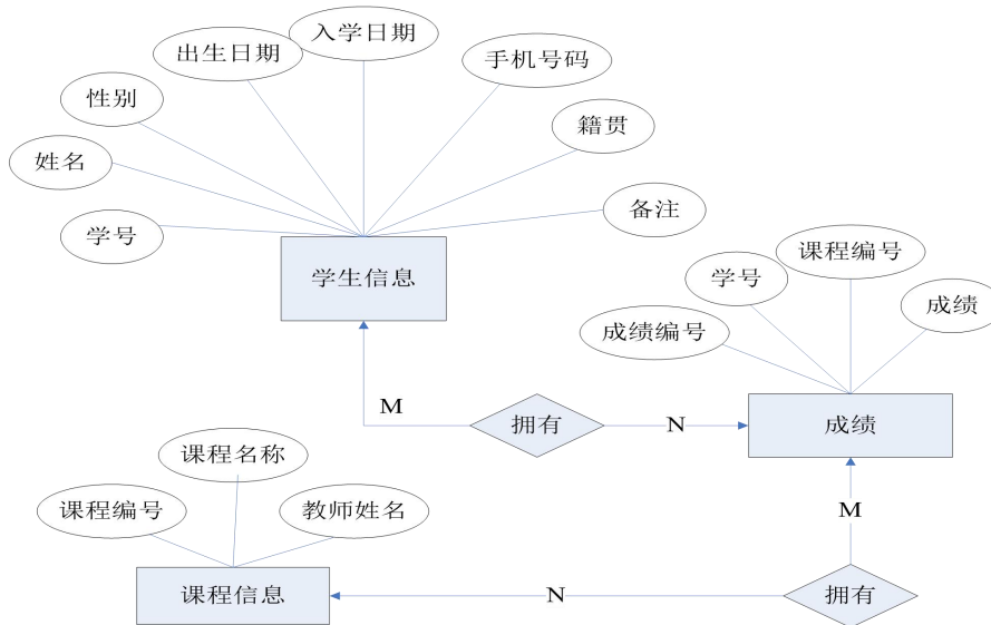
图 2.1.1 E-R 图
