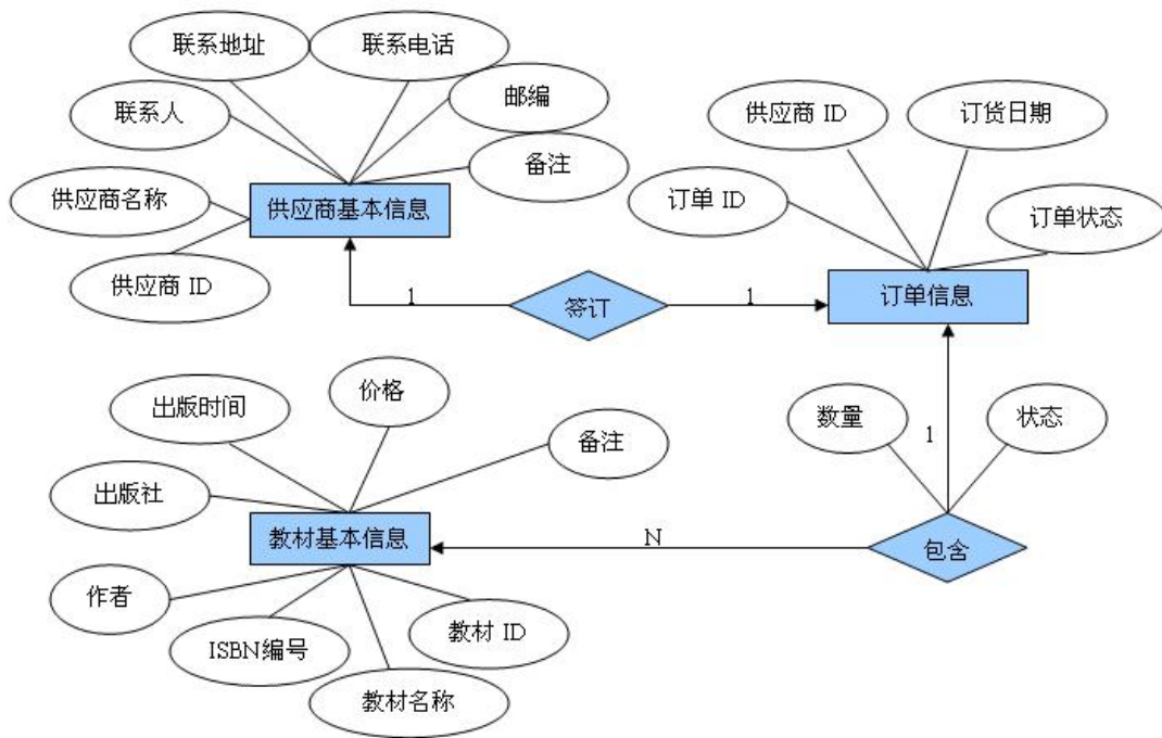
图 2.2.1 E-R 图
