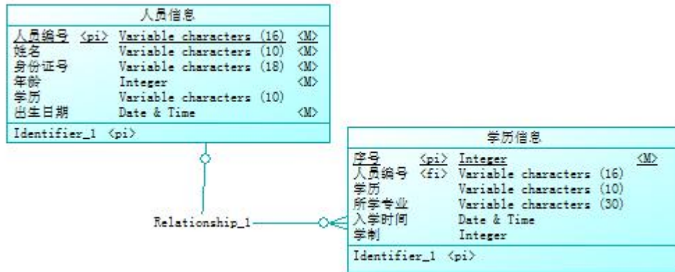
图 2.7.2 逻辑数据模型
