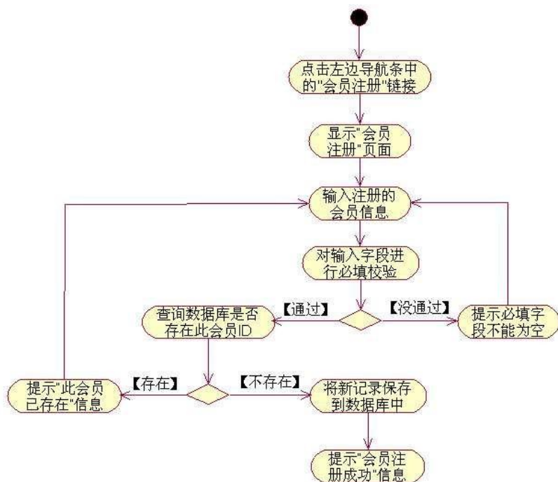
图 1.25.4 会员注册活动图
