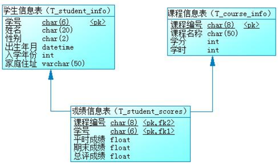
图 2.4.3 物理数据原型
