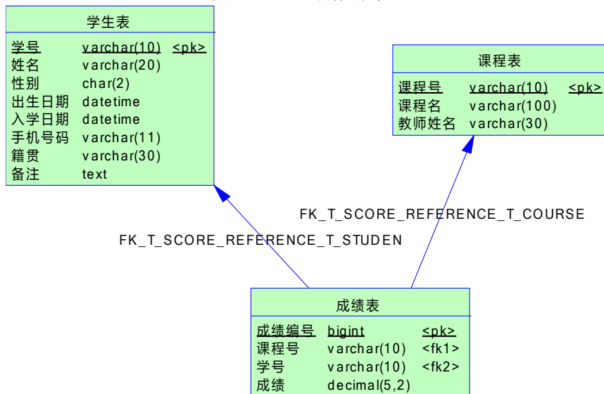
图 2.1.3 物理数据原型
