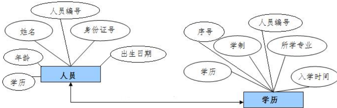
图 2.7.1 E-R 图
