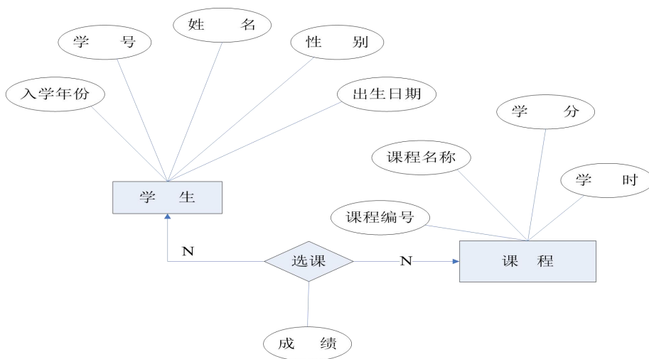
图 2.4.1 E-R 图
