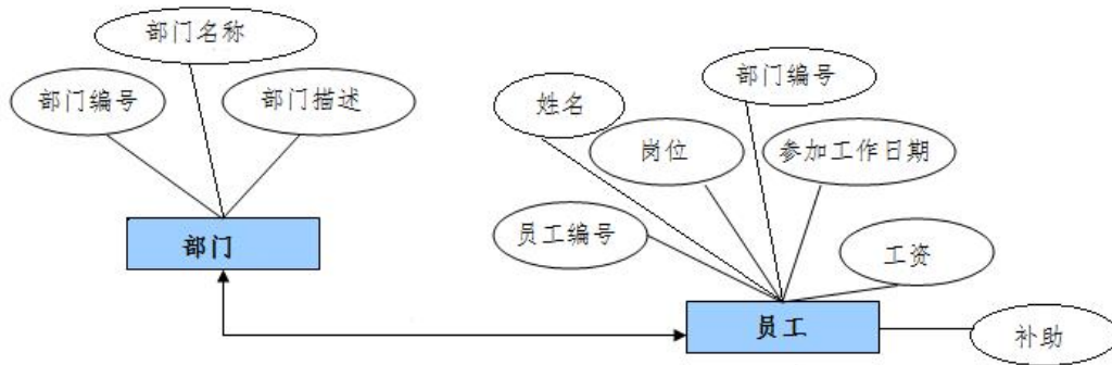
图 2.8.1 E-R 图
