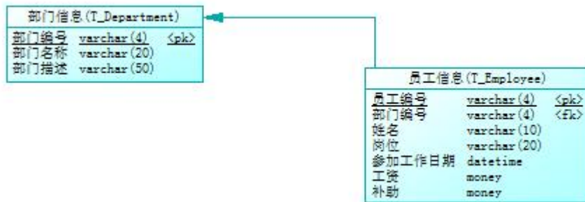
图 2.8.3 物理数据原型
