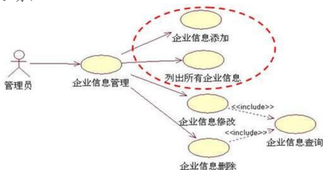
图 1.2.3 企业信息管理模块用例图
