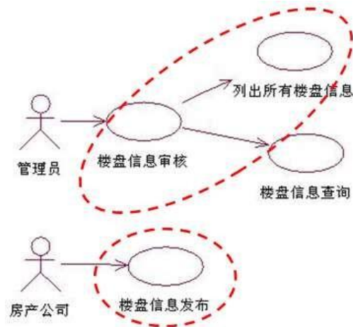
图 3.7.3 易居房产信息网楼盘发布模块用例图
