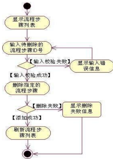
图 3.4.5 删除流程步骤信息活动图
